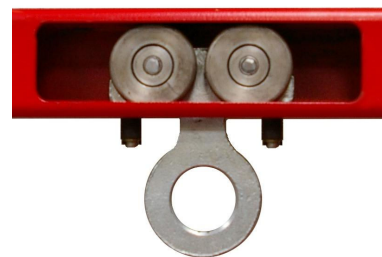
Carretilla polipasto
