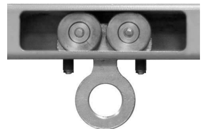
Carretilla polipasto
